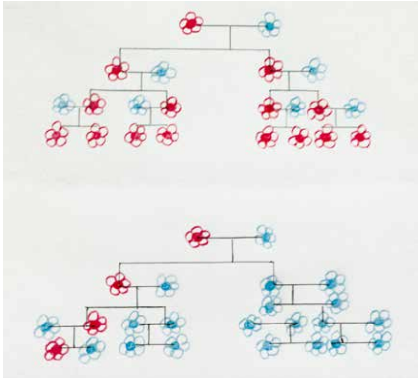
Oben: Die Vererbung mit Gene Drive führt im Unterschied zu der Vererbung nach dem Mendelschen Gesetzen (unten) dazu, dass nach wenigen Generationen sich eine Eigenschaft komplett durchsetzt. Wenn diese Eigenschaft z.B. ist, dass nur weibliche Organismen überleben, stirbt eine Art aus.
